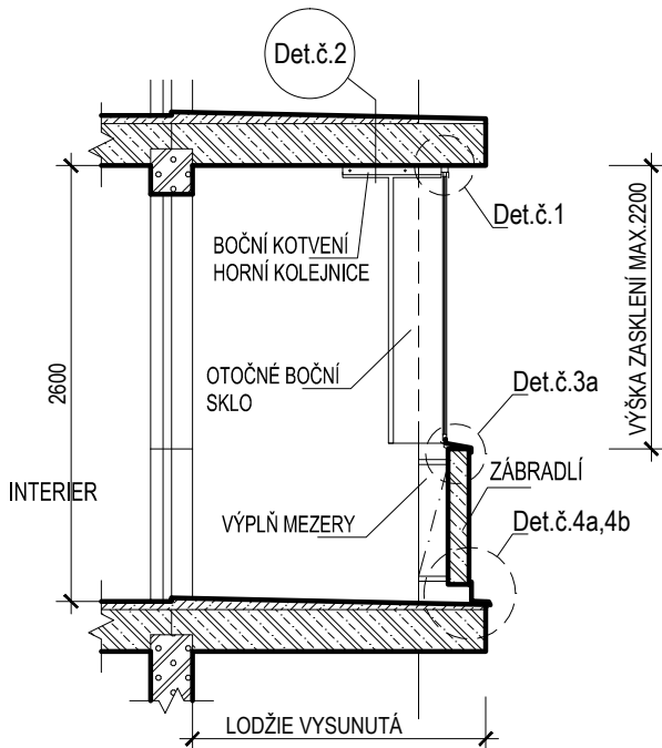
ŘEZ A M1:50
