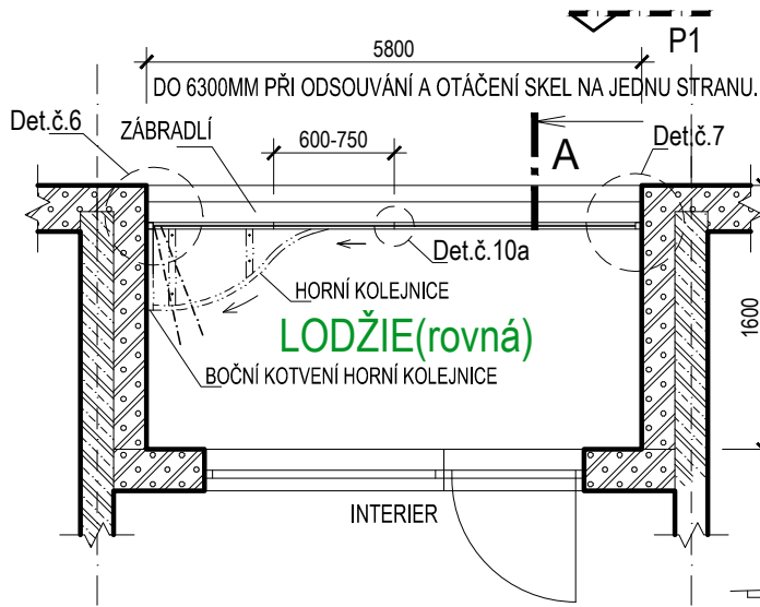
POHLED M1:50
