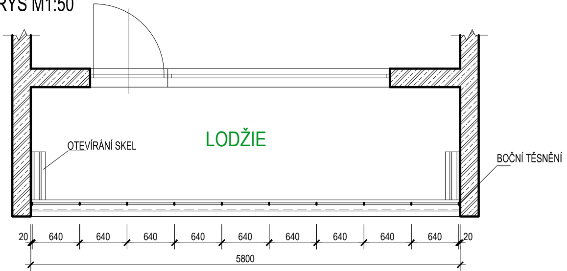
POHLED M1:50
