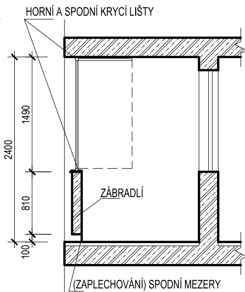
ŘEZ A
